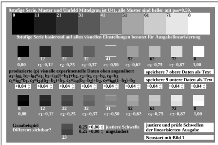
igb81-4a, Bild 4, produziere (p) Sehschwelle (+0,04?) von 9 Stufen; alle gleich?, \gamma_{rel}=0,75
