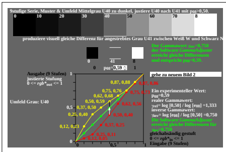
igb81-1a, Bild 1, produziere (p) gleiche Differenz zwischen Schwarz N – Weiß W, \gamma_{rel}=0,75
