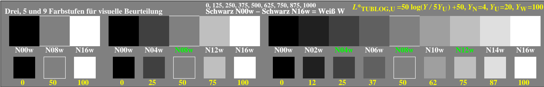
ggv70-5n, Prüfmuster: 3, 5 und 9 Farbstufen, greu=0,500, expu=1,000, expa=1,000
