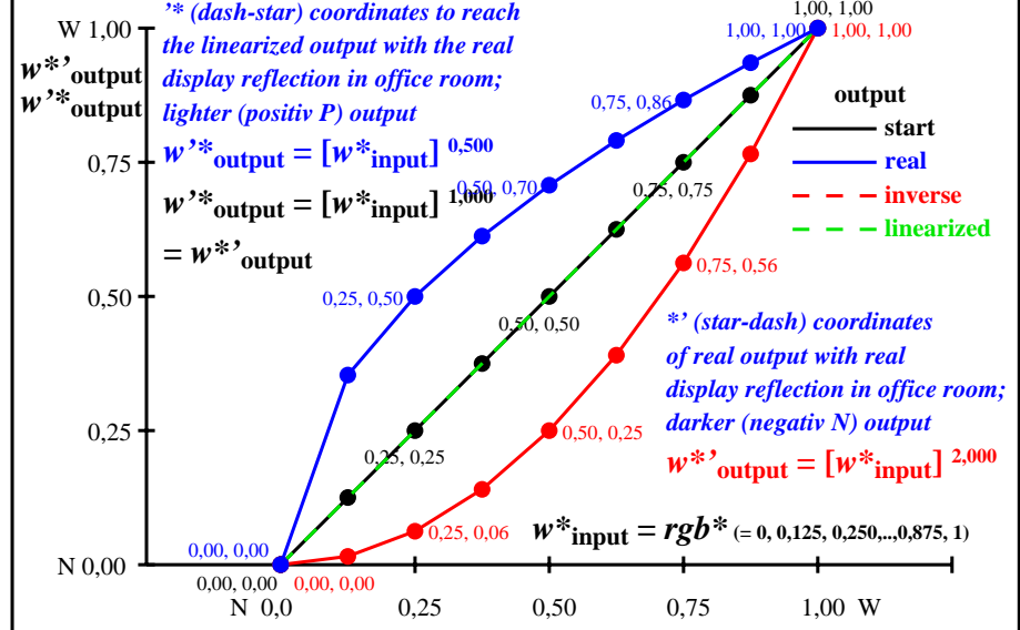
gew71-3n
