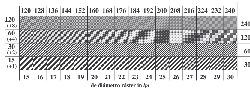
TS781-3, Fig. C5We: Elemento E: Trama línea menores de 45° (o 135°) grados; PS operator: rgb/cmy0
