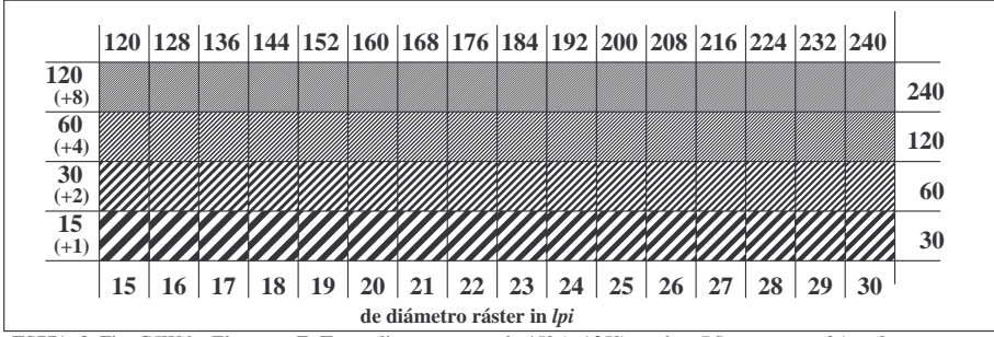
TS771-3, Fig. C5Wde: Elemento E: Trama línea menores de 45° (o 135°) grados; PS operator: rgb/cmy0
