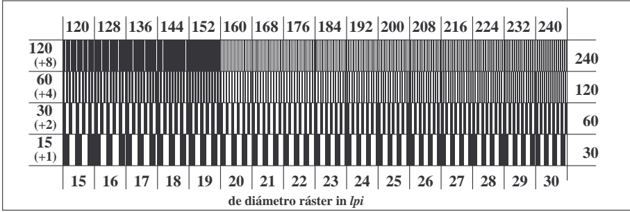
TS771-5, Fig. C6Wde: Elemento F: Trama línea menores de 90° (o 0°) grados; PS operator: rgb/cmy0
