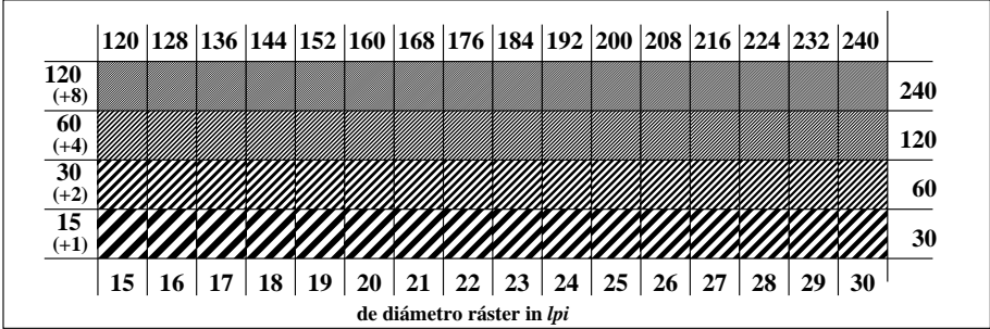
TS761-3, Fig. C5W-: Elemento E: Trama línea menores de 45° (o 135°) grados; PS operator: rgb/cmy0
