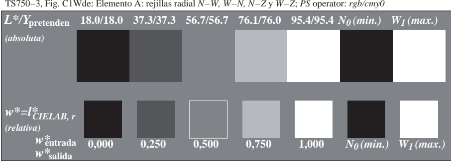
TS750-5, Fig. C2Wde: Elemento B: 5 equidistante L^* pasos de gris + N_0 + W_1 ; PS operator: rgb/cmy0
