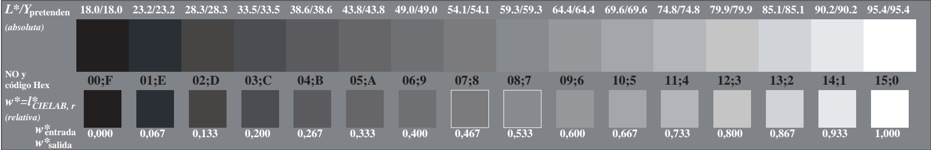
TS750-7, Fig. C3Wde: Elemento C: 16 equidistante L^* pasos de gris; PS operator: rgb/cmy0
