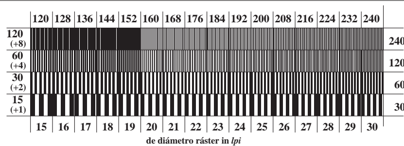
TS751-5, Fig. C6Wdd: Elemento F: Trama línea menores de 90° (o 0°) grados; PS operator: rgb/cmy0
