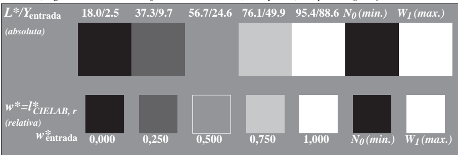
TS750-5, Fig. C2We: Elemento B: 5 equidistante L^* pasos de gris + N_0 + W_1 ; PS operator: rgb/cmy0
