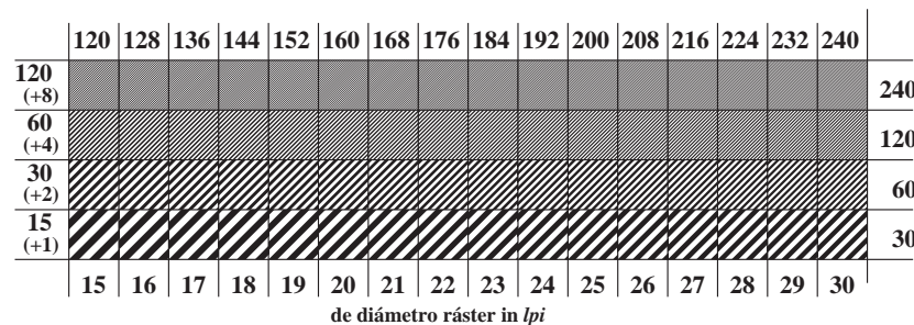
TS751-3, Fig. C5We: Elemento E: Trama línea menores de 45° (o 135°) grados; PS operator: rgb/cmy0
