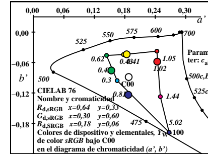
2-000530-L0 TS481-3N_6
