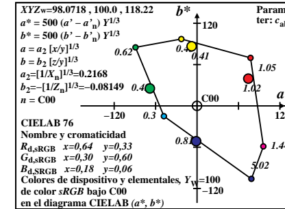
2-000530-L0 TS481-6N_6
