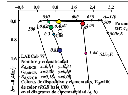
2-000530-L0 TS481-2N_6
