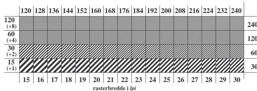
TN771-3, Figur C5Wde: Element E: Linjeraster med 45° (eller 135°); PS operator: rgb/cmy0
