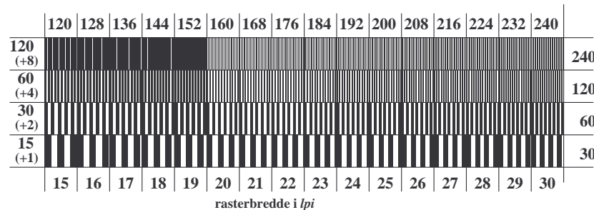
TN771-5, Figur C6Wde: Element F: Linjeraster med 90° (eller 0°); PS operator: rgb/cmy0
