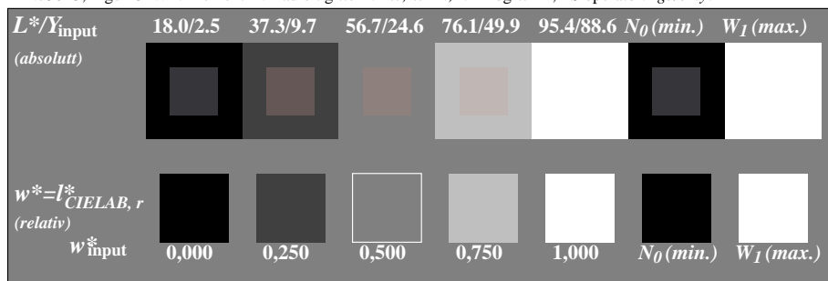
TN750-5, Figur C2W-: Element B: 5 visuelle ekvidistante L^* -gråtrinn + N_0 + W_1 ; PS operator: rgb/cmy0
