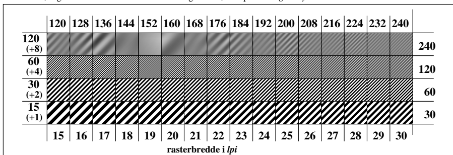
TN751-3, Figur C5W-: Element E: Linjeraster med 45° (eller 135°); PS operator: rgb/cmy0
