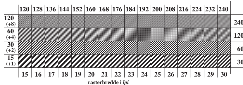
TN741-3, Figur C5We: Element E: Linjeraster med 45° (eller 135°); PS operator: rgb/cmy0
