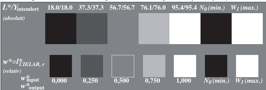
TN740-5, Figur C2Wdd: Element B: 5 visuelle ekvidistante L^* -gråtrinn + N_0 + W_I ; PS operator: rgb/cmy0
