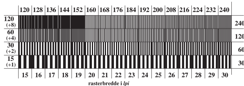
TN741-5, Figur C6Wdd: Element F: Linjeraster med 90° (eller 0°); PS operator: rgb/cmy0
