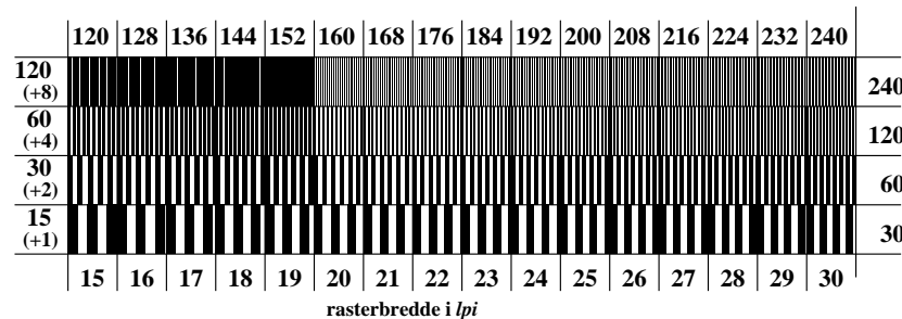
TN721-5, Figur C6Wd: Element F: Linjeraster med 90° (eller 0°); PS operator: rgb/cmy0
