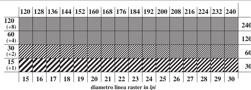
TI791-3, Fig. C5Wd: Elemento E: Linea raster a 45° (o 135°) gradi; PS operator: rgb/cmy0
