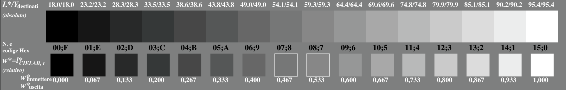
TI720-7, Fig. C3Wde: Elemento C: 16 equidistante L^* grigio passi; PS operator: rgb/cmy0
