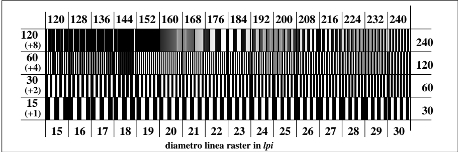
TI721-5, Fig. C6We: Elemento F: Linea raster a 90° (o 180°) gradi; PS operator: rgb/cmy0
