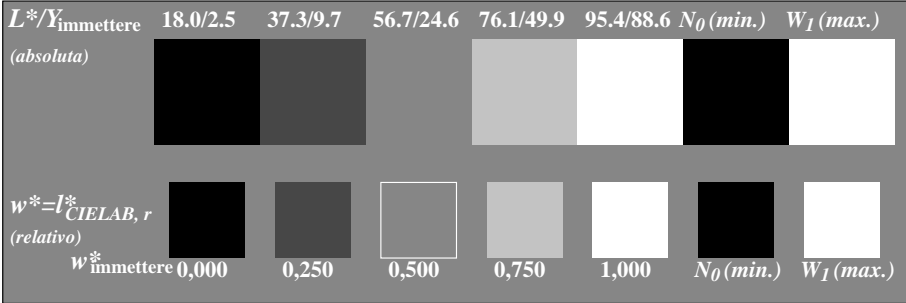
TI720-5, Fig. C2We: Elemento B: 5 equidistante L^* grigio passi + N_0 + W_1 ; PS operator: rgb/cmy0
