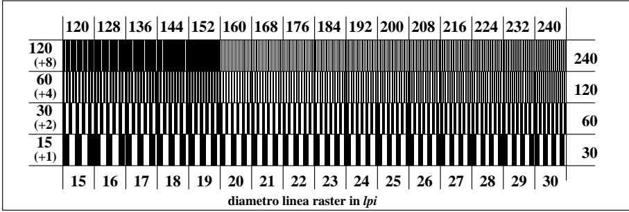
TI1721-5, Fig. C6Wdd: Elemento F: Linea raster a 90° (o 180°) gradi; PS operator: rgb/cmy0
