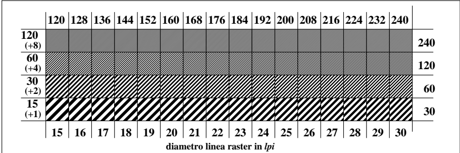
TI721-3, Fig. C5We: Elemento E: Linea raster a 45° (o 135°) gradi; PS operator: rgb/cmy0
