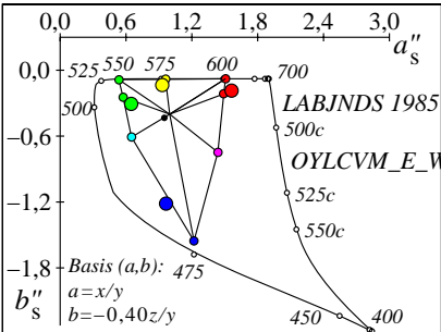
JG570-7, Farben in (a''_s, b''_s) Farbtafel
