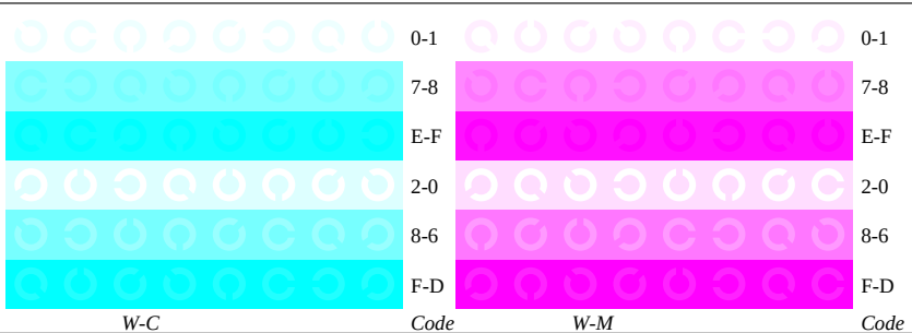
Fig. B6: anillos de Landolt W-C y W-M ; PS operator: olv * setrgbcolor / w * setgray
