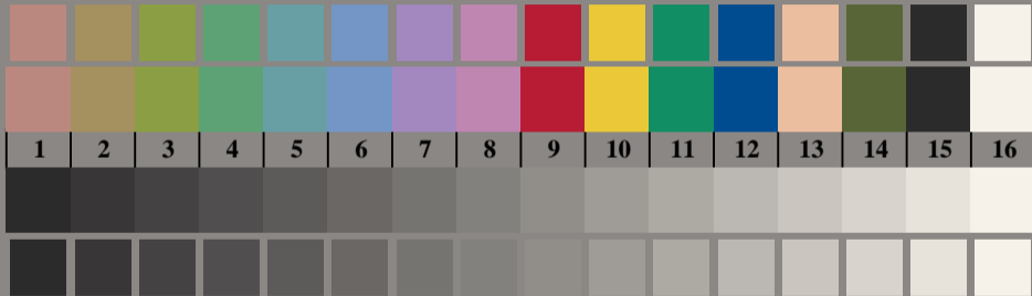
Fig. D3: 14 CIE test couleurs et 2 + 16 paliers de gris (sf); PS opérateur : LAB* setcolor
