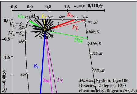
DEO60-4A
