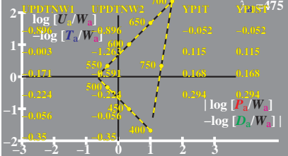
WG991-6, Änderung von PDT (LMS) beim Farbsehen; Adaptation
