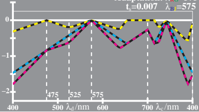
WG971-3, Änderung von PDT (LMS) beim Farbsehen; Adaptation
