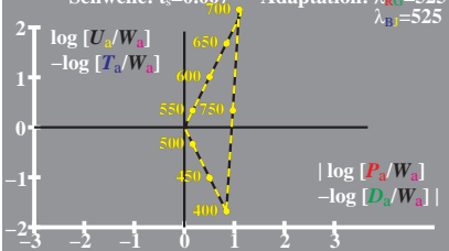
WG961-2, Änderung von PDT (LMS) beim Farbsehen; Adaptation
