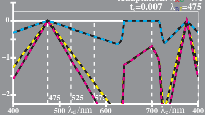
WG941-5, Änderung von PDT (LMS) beim Farbsehen; Adaptation
