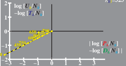
WG941-2, Änderung von PDT (LMS) beim Farbsehen; Adaptation
