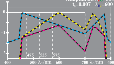
WG931-7, Änderung von PDT (LMS) beim Farbsehen; Adaptation
