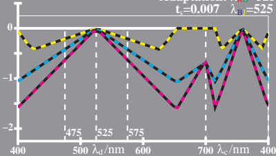
WG911-1, Änderung von PDT (LMS) beim Farbsehen; Adaptation
