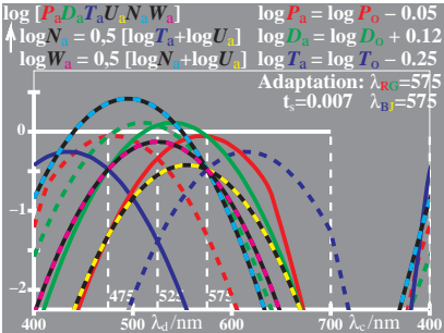
WG910-3, Änderung von PDT (LMS) beim Farbsehen; Adaptation
