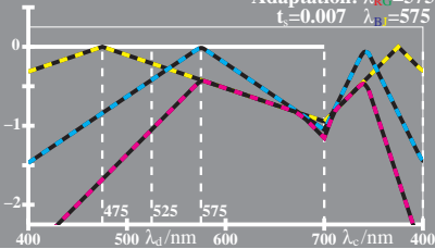
WG901-3, Änderung von PDT (LMS) beim Farbsehen; Adaptation
