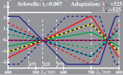
WG900-2, Änderung von PDT (LMS) beim Farbsehen; Adaptation
