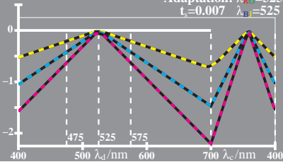
WG891-1, Änderung von PDT (LMS) beim Farbsehen; Adaptation
