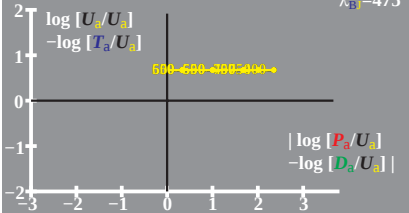
WG881-2, Änderung von PDT (LMS) beim Farbsehen; Adaptation
