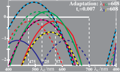
WG870-7, Änderung von PDT (LMS) beim Farbsehen; Adaptation
