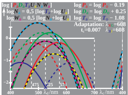
WG860-7, Änderung von PDT (LMS) beim Farbsehen; Adaptation
