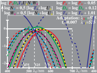
WG840-3, Änderung von PDT (LMS) beim Farbsehen; Adaptation
