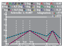
WG831-7. Änderung von PDT (LMS) beim Farbsehen, Adaptation
