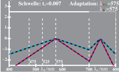
WG831-7, Änderung von PDT (LMS) beim Farbsehen; Adaptation
