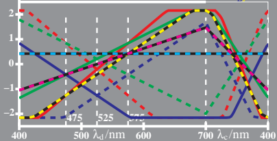
WG810-8, Änderung von PDT (LMS) beim Farbsehen; Adaptation
