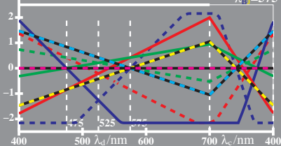
WG801-7, Änderung von PDT (LMS) beim Farbsehen; Adaptation
