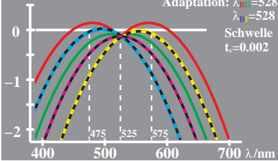
WG791-3, Änderung von PDT (LMS) beim Farbsehen; Adaptation
