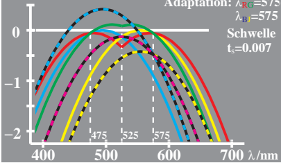
WG790-5, Änderung von PDT (LMS) beim Farbsehen; Adaptation
