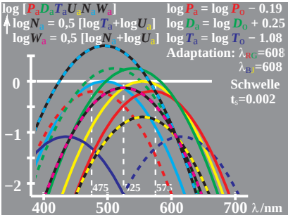
WG781-7, Änderung von PDT (LMS) beim Farbsehen; Adaptation
