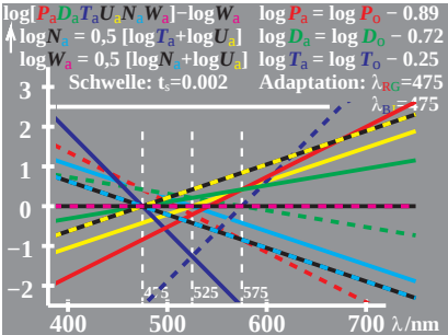
WG781-2, Änderung von PDT (LMS) beim Farbsehen; Adaptation
