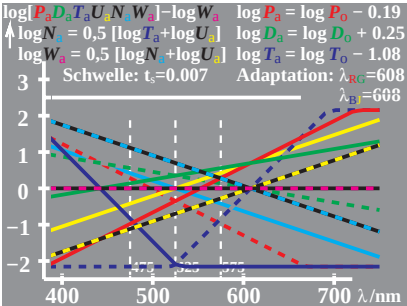
WG780-8, Änderung von PDT (LMS) beim Farbsehen; Adaptation
