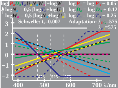
WG780-6, Änderung von PDT (LMS) beim Farbsehen; Adaptation
