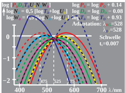
WG780-3, Änderung von PDT (LMS) beim Farbsehen; Adaptation
