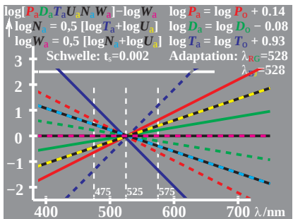
WG771-4, Änderung von PDT (LMS) beim Farbsehen; Adaptation
