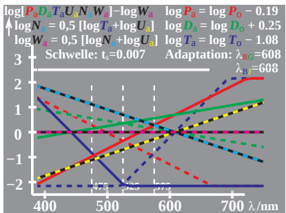
WG770-8, Änderung von PDT (LMS) beim Farbsehen; Adaptation
