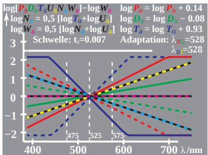
WG770-4, Änderung von PDT (LMS) beim Farbsehen; Adaptation
